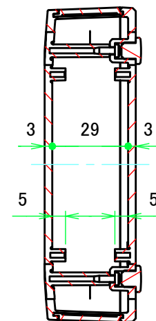
A-A ( 1 : 2 )
