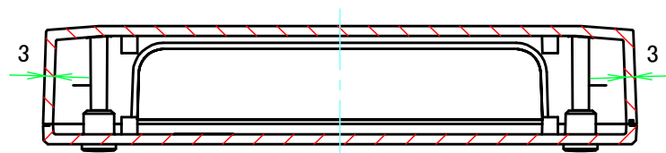
B-B ( 1 : 2 )
